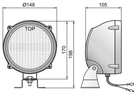
Размеры
