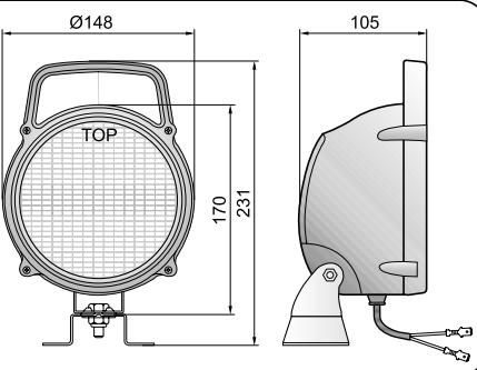
Размеры
